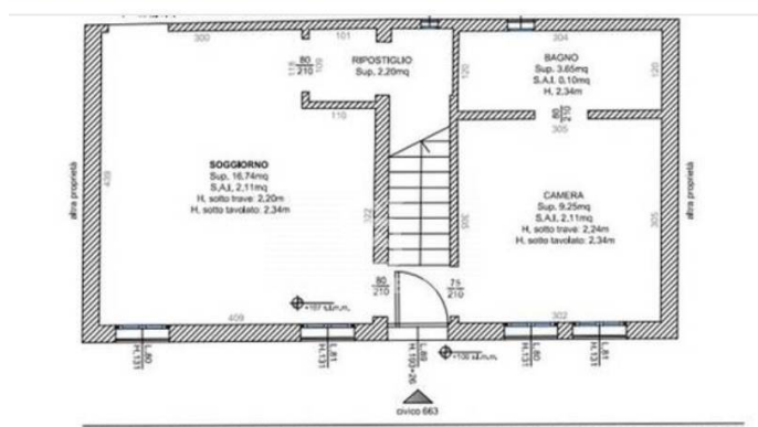
STATO DI PROGETTO Planimetria piano terra scala 1:50
