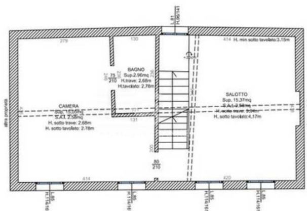
STATO DI PROGETTO Planimetria piano secondo scala 1:50
