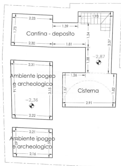
PIANTA AMBIENTI INTERRATI superficie netta 27,5 mq
