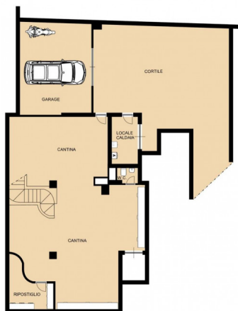
PIANTA PIANO CANTINATO
