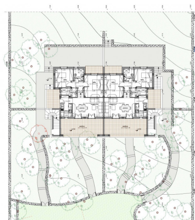
Pianta Piano Terra rapp. 1:100
