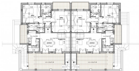
Pianta Piano Primo rapp. 1:100
