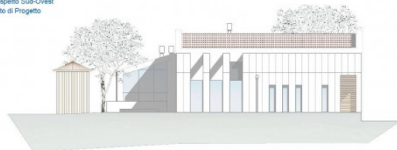
Prospetto Sud-Ovest Stato di Progetto
