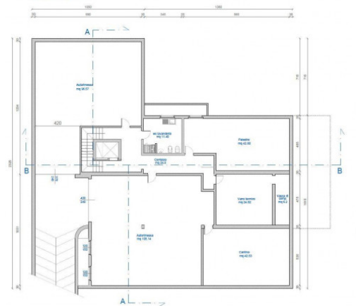
PIANTA PIANO INTERRATO Stato di Progetto
