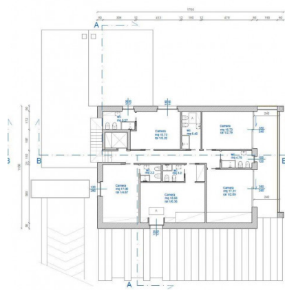
PIANTA PIANO PRIMO Stato di Progetto
