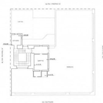
PIANO SECONDO ESISTENTE Rapp. 1:100
