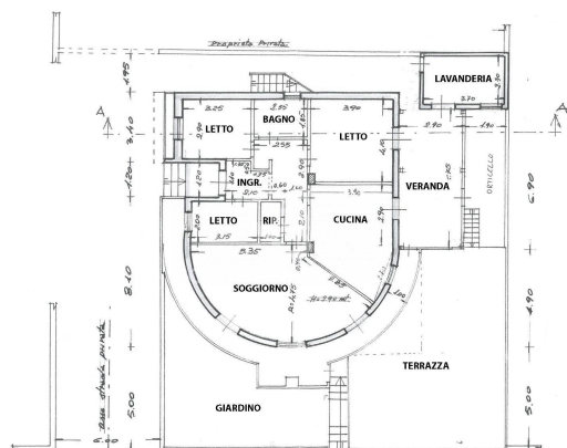
PLANIMETRIA PIANOTERRA
