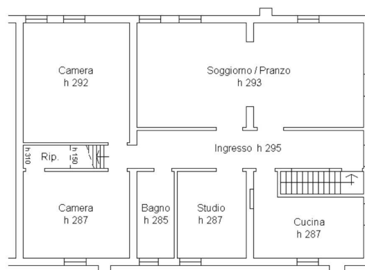
PIANO SECONDO
