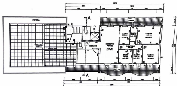
PIANTA DEL PIANO QUARTO
