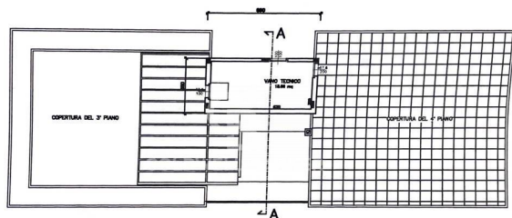
PIANTA DELLA COPERTURA
