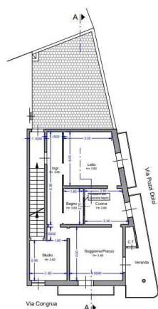
PIANO PRIMO - R. 1/ 100
