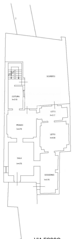
VIA FOSSO PIANO TERRA
