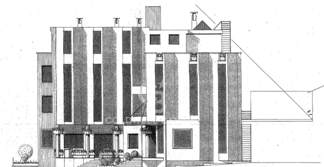
PROSPETTO
