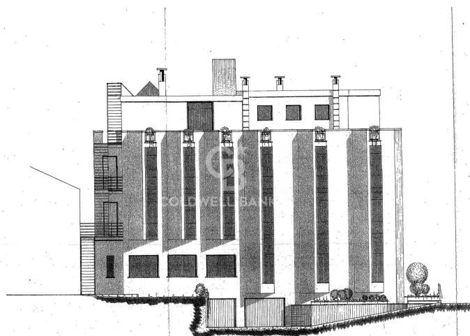
PROSPETTO LATERALE - OVEST
