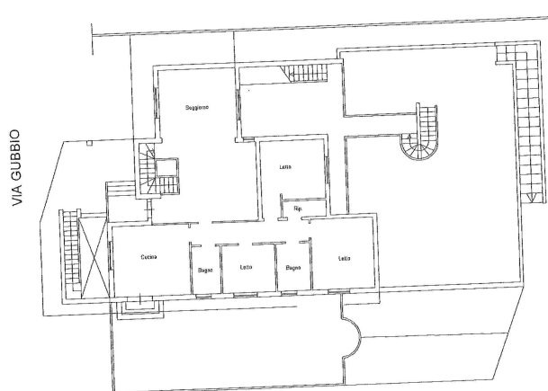
PIANO RIALZATO H= 3,05
